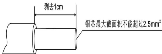
图 2-5 电源线的处理要求
