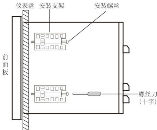
图 2 安装图
