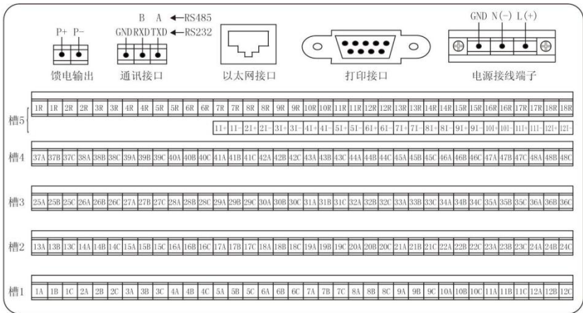
配线说明
