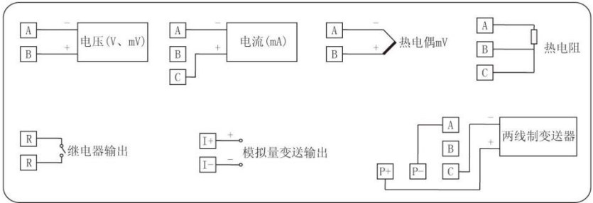
图 3 接线端子
