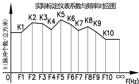
图 15 实际标定仪表系数与频率对应图
