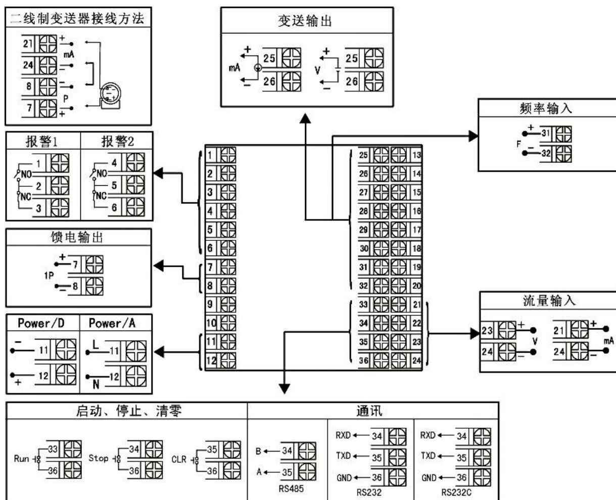
图 4 无补偿流量接线图
