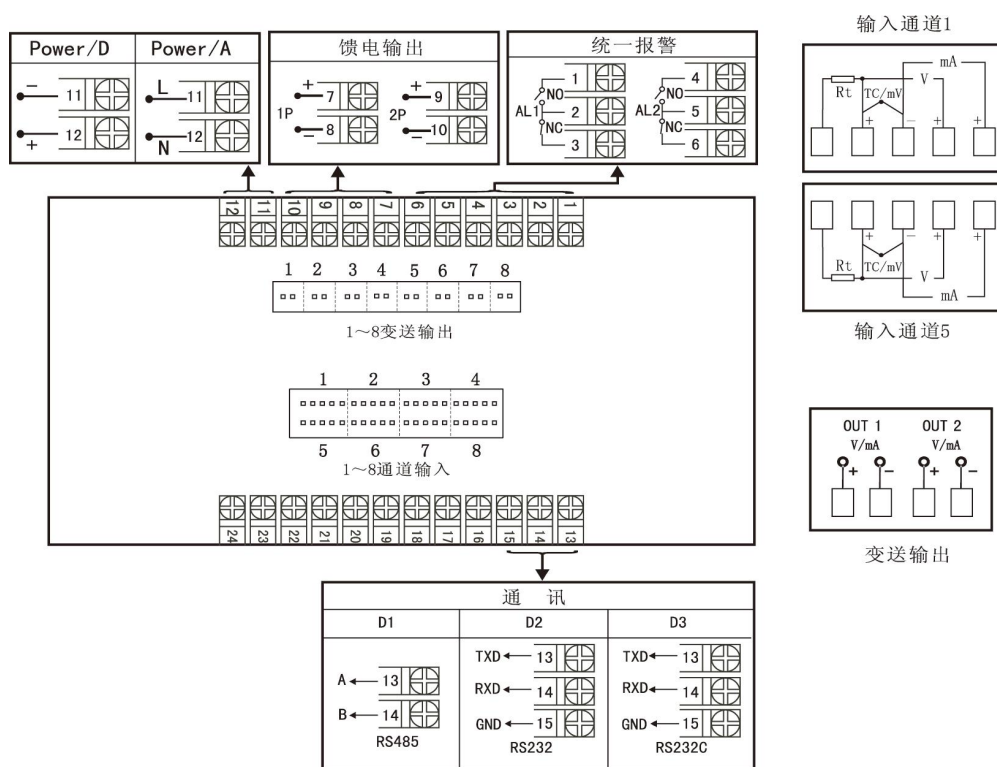
图 7 C 型分别变送接线图
