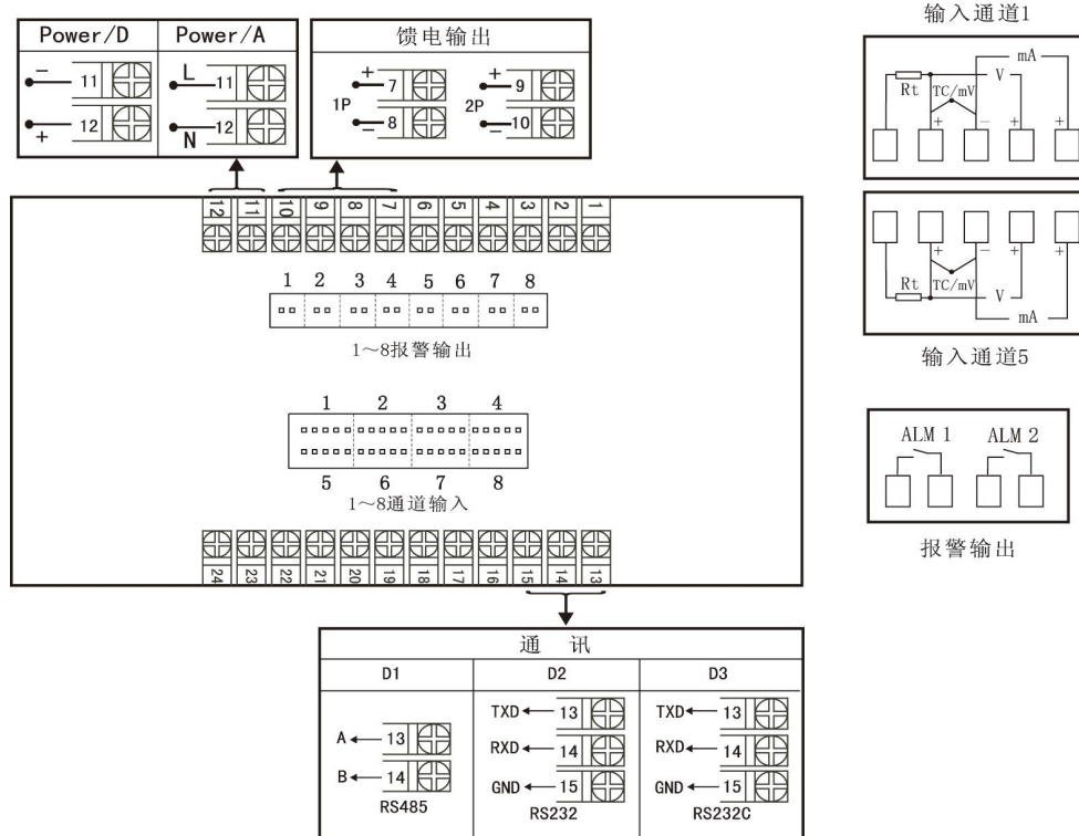
图 6 C 型分别报警接线图
