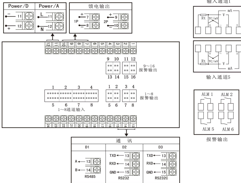
图 4 A、B 型分别报警接线图
