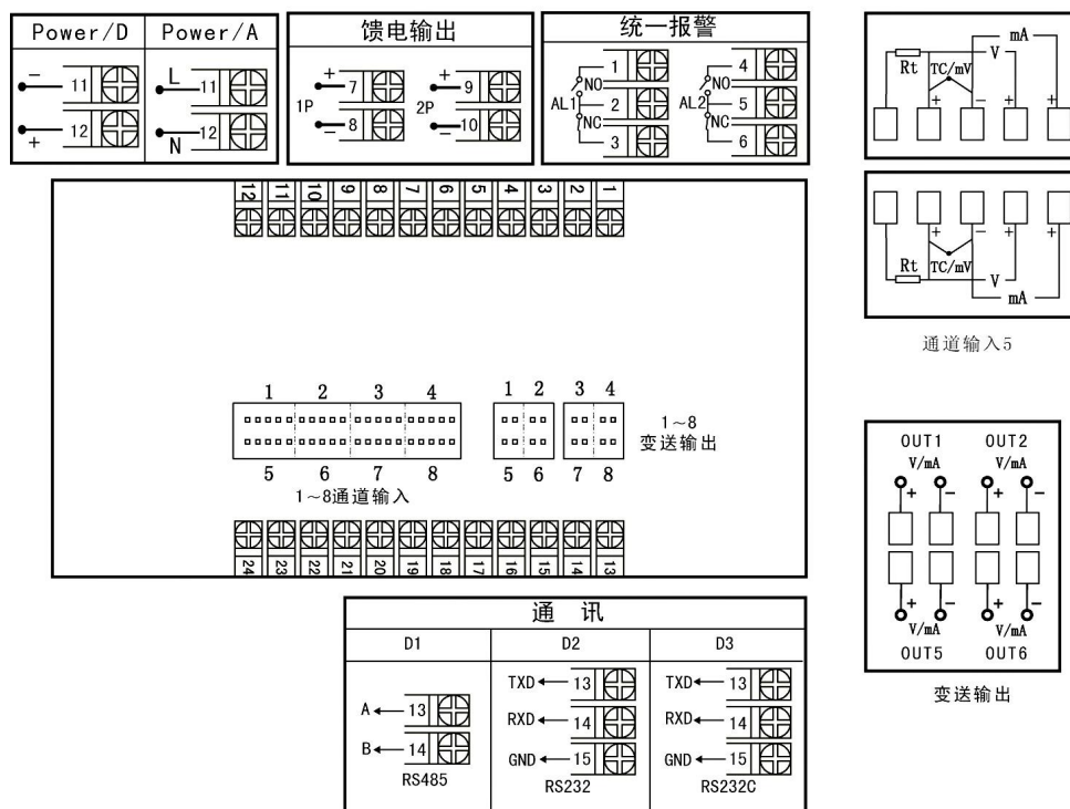
图 5 A、B 型分别变送接线图
