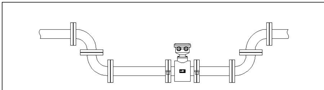
图 4.2.1 防负压安装
