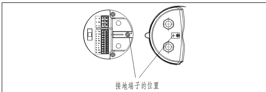
图 5.5.1 转换器接地
