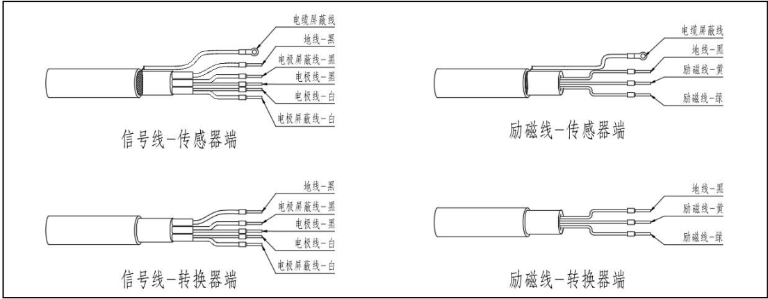
图 5.2.2 标准电缆示意图
